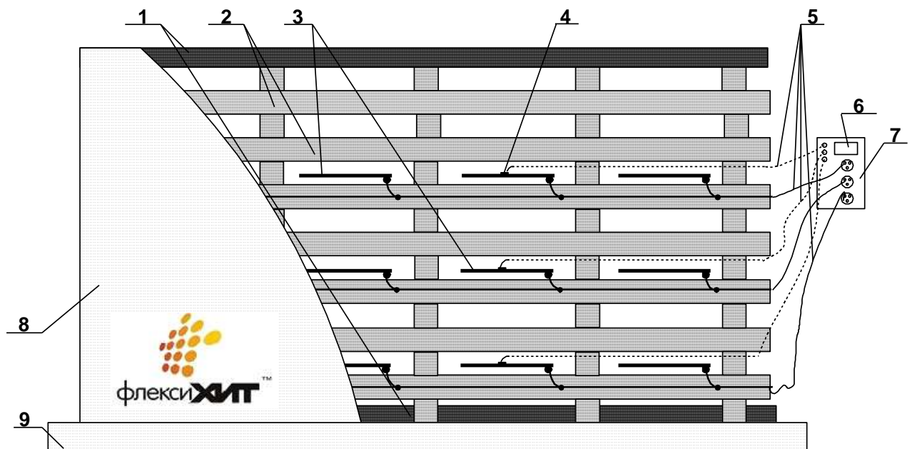
Рис. 3: 1. Теплоизолятор; 2. Древесина; 3. Нагреватель; 4. Термодатчик; 5. Электропровода; 6. Трехканальный терморегулятор; 7. Электрощит; 8. Конденсирующая оболочка, с отражающим покрытием; 9. Жесткое основание.
